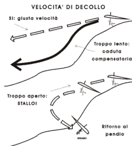
Figura 5-16. La velocità del veicolo di decollo deve consentire uno stacco lineare: decollando troppo lentamente il delta effettua una caduta compensatoria per guadagnare velocità, oppure stalla tornando verso il
