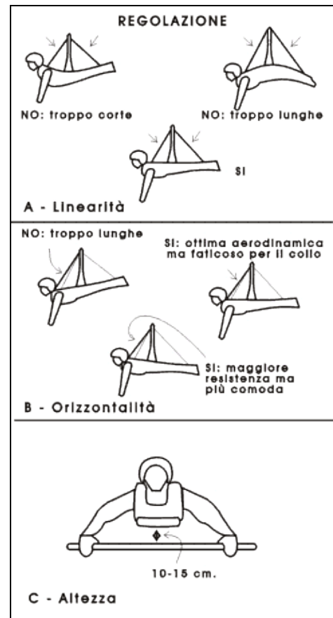
Figura 5-8. Le tre fasi della regolazione di un'imbragatura: linearità, orizzontalità e distanza dalla barra di controllo.
