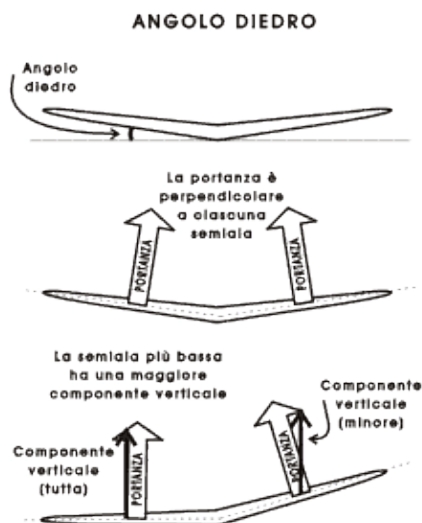
Figura 5-35. L'angolo diedro conferisce stabilità laterale generando differenze di portanza.
