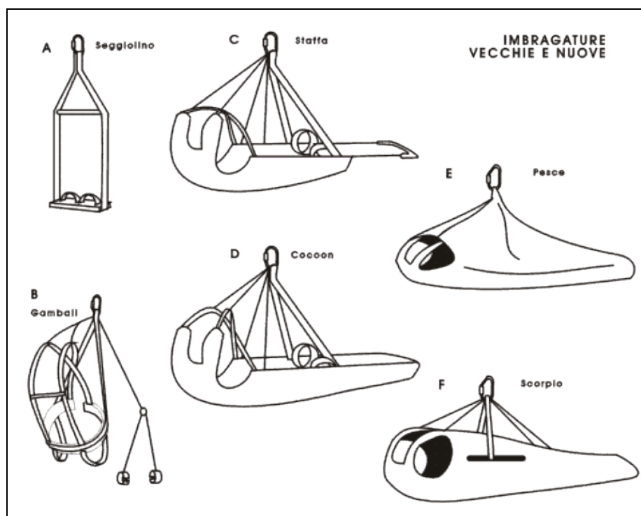
Figura 5-7. Modelli di imbragatura
