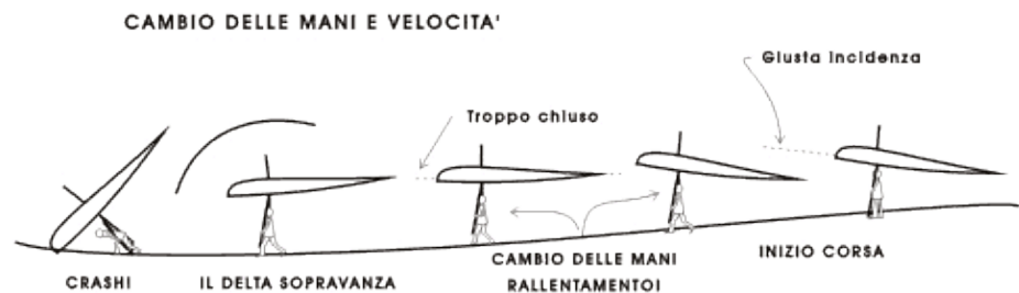
Figura 5-15. L'errato (ed involontario) rallentamento al momento del cambio delle mani, determina un'accelerazione del deltaplano che ci sopravanza: è necessario evitare il rallentamento e mantenere la progressiva della corsa.
