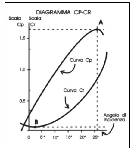
Figura 3-16. Diagramma Cp-Cr.
