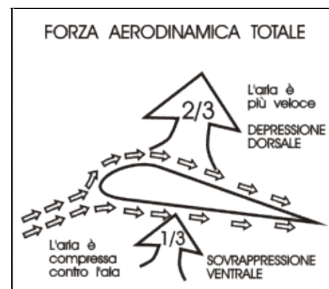
Figura 3-10. Genesi della Forza Aerodinamica Totale, che rende possibile il volo.
