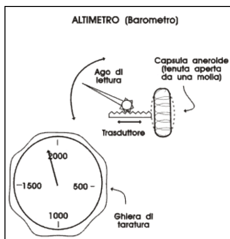
Figura 7-2. L'altimetro (barometro) permette di leggere le variazioni di pressione come variazioni di altitudine.
