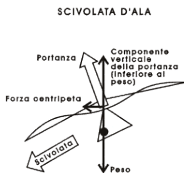
Figura 5-24. La scivolata d'ala per mancata (od insufficiente) cabrata.
