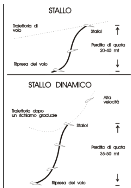
Figura 3-20. Il recupero da una posizione di stallo richiede una quota anche notevole (maggiore in seguito a stallo dinamico).
