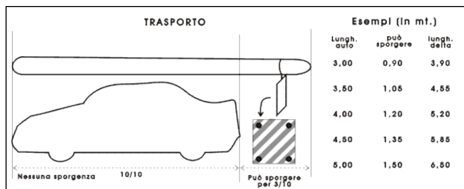
Figura 5-6. La legge italiana pone precise limitazioni al trasporto di carichi sporgenti sugli autoveicoli.
