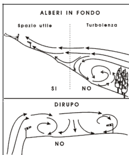
Figura 6-17. Gli alberi in fondo al terreno di decollo ne limitano la sfruttabilità, per le turbolenze che generano.
