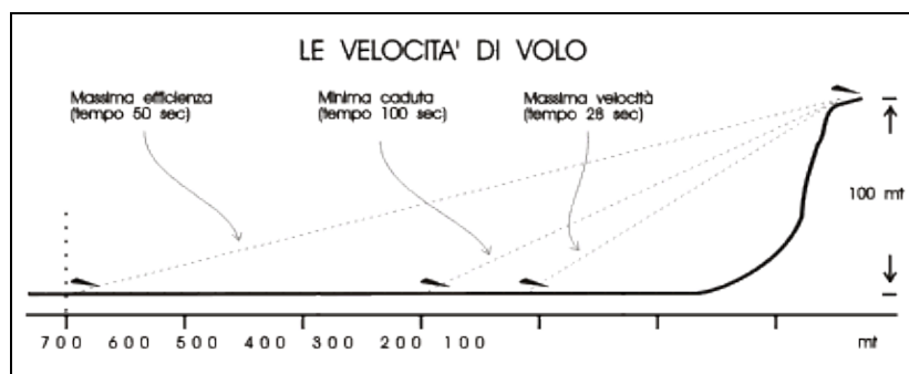
Figura 3-15. Tempi di volo e distanze compiute volando alle diverse velocità.
