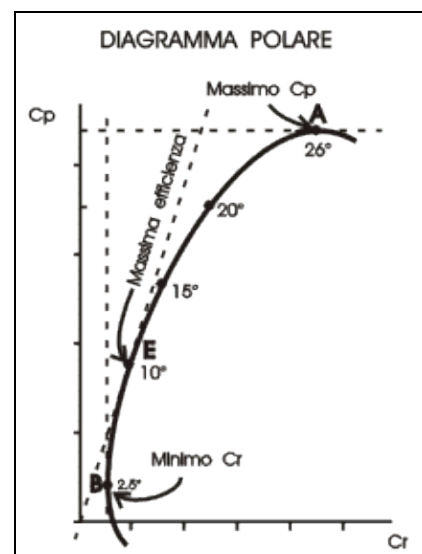
Figura 3-17. Diagramma Polare.
