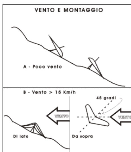
Figura 5-5. Posizioni per il montaggio sul pendio debole (A) o con vento sostenuto (B).
