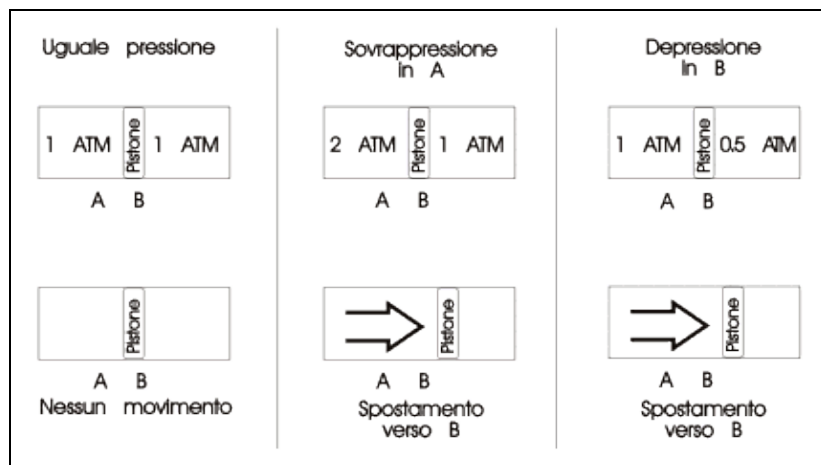
Figura 3-3. Ciò che determina lo spostamento del separatore mobile è la differenza di pressione tra A e B: ciò può essere ottenuto sia determinando una sovrappressione in A sia riducendo la pressione in B.
