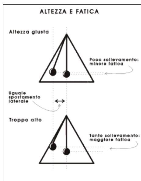
Figura 5-9. Un aggancio troppo alto richiede un maggior sforzo per ottenere lo stesso spostamento laterale del peso. Un aggancio troppo alto rende faticosa e difficile la manovra , (oltre che per i motivi esposti in figura 5-9, anche perché si è costretti a pilotare con le braccia distese), ma un aggancio troppo basso comporta il rischio che la sacca del paracadute , strofinando contro la barra di controllo, si apra con conseguenze anche molto gravi, per noi e per l'apparecchio.
