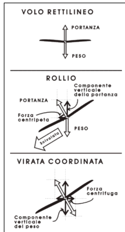
Figura 3-22. La cabrata ha l'effetto di riequilibrare le forze impedendo la scivolata d'ala.
