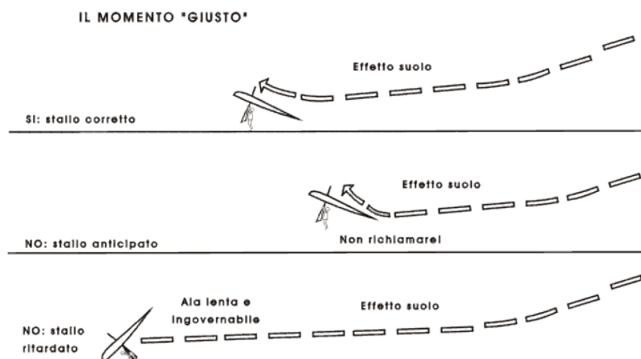
Figura 5-16. Stallando troppo presto il delta si rialza, ritardando esso non si ferma, ma spaccia fino al suolo.
