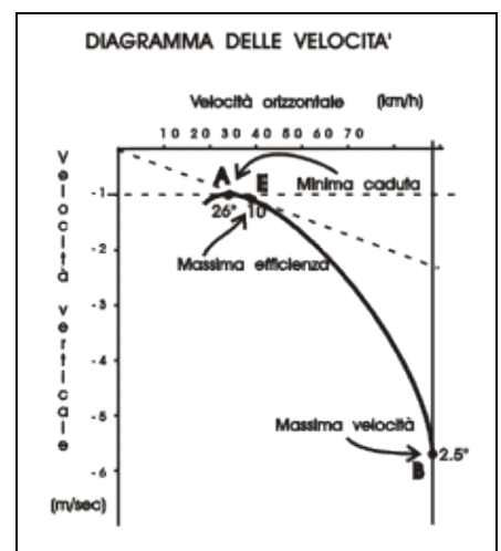
Figura 3-18. Diagramma delle Velocità.
