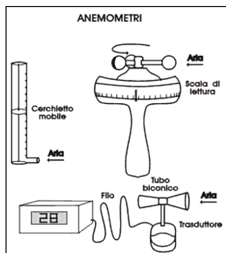
Figura 7-5. Alcuni tipi di anemometri utilizzati nel Volo Libero.
