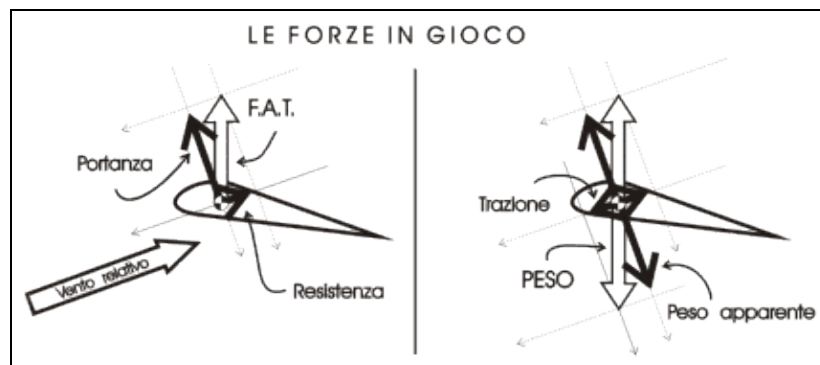
Figura 3-11. Le due forze che compongono la F.A.T. (portanza e resistenza) sono, nel volo planato uniforme, in perfetto equilibrio con le due che compongono il PESO (peso apparente e trazione).
