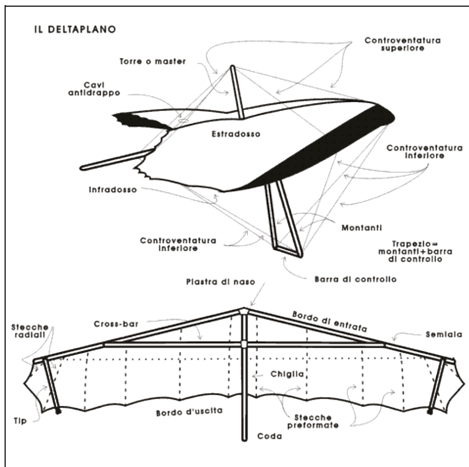
Figura 5-1. Deltaplano e corretta denominazione delle sue parti: come si può notare alcuni termini sono presi "pari pari" dall'aeronautica classica mentre altri sono tipici di questo apparecchio. L'insieme dei cavi viene detto controventatura (superiore ed inferiore) mentre le due superfici alari costituiscono l'estradosso (sopra) e l'infradosso (sotto).
