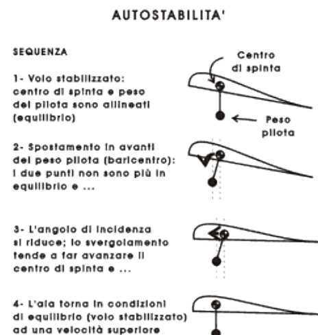
Figura 5-34. Quando il baricentro si sposta in avanti, il centro di spinta (per effetto dello svergolamento) tende a spostarsi in avanti anch'esso, ristabilendo un equilibrio.
