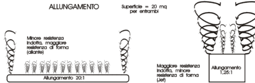
Figura 3-24. L'allungamento riduce la resistenza indotta: tale effetto è particolarmente rilevante per gli apparecchi che volano a basse velocità.
