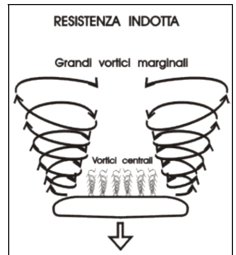
Figura 3-14. Resistenza indotta: è massima alle basse velocità.
