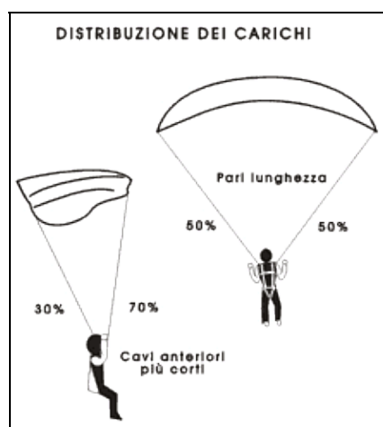
Figura 6-24. La distribuzione dei carichi dipende direttamente dalla lunghezza dei cordoni.
