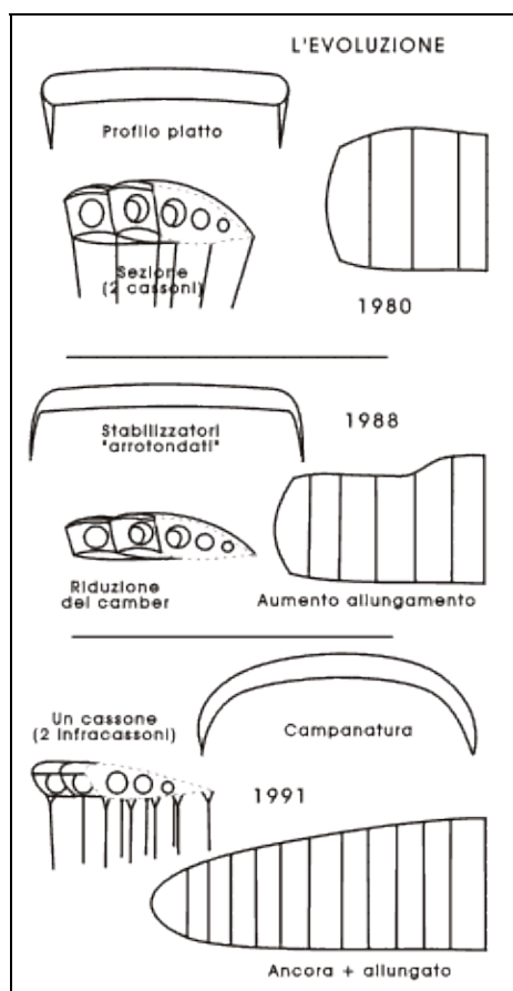
Figura 6–2. IRappresentazione schematica (e leggermente enfatizzata) dell'evoluzione del parapendio negli anni.
