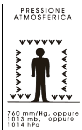
Figura 4-1. La pressione atmosferica esercita il suo effetto su tutte le superfici.
