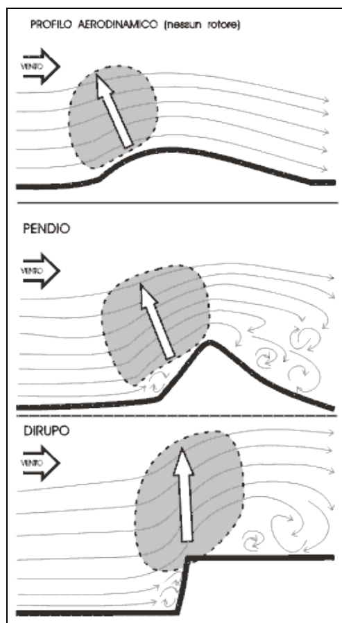
Figura 4–16. Use la montagna non ha un profilo "alare", in presenza di vento si formano rotori (R), sia a valle che a monte della zona di ascendenza.
