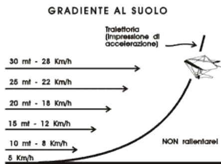
Figura 5-27. Il gradiente di vento dà la sensazione di un'improvvisa accelerazione: evitare un pericoloso rallentamento.
