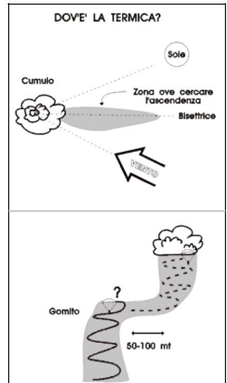
Figura 8-5. La zona di ascendenza deve essere ricercata sulla bisettrice dell'angolo che il cumulo forma con il sole e con la direzione del vento. A volte le termiche formano veri e propri gomiti, e proseguono sottovento.
