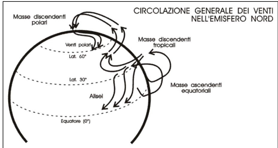
Figura 4-25. La circolazione generale delle masse d'aria risente del moto rotatorio terrestre: così i venti polari provengono anche da est, mentre quelli delle zone intermedie hanno una componente occidentale.
