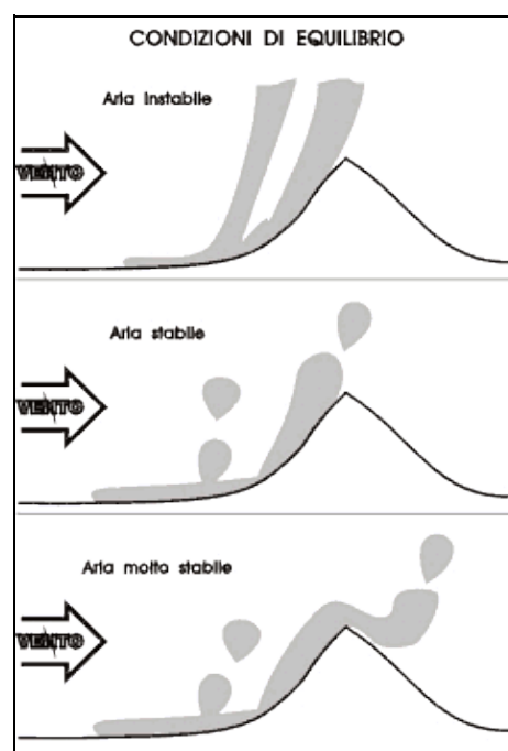
Figura 8-3. Naturalmente la stabilità dell'aria è determinante: aria instabile=termiche frequenti e che raggiungono quote elevate.
