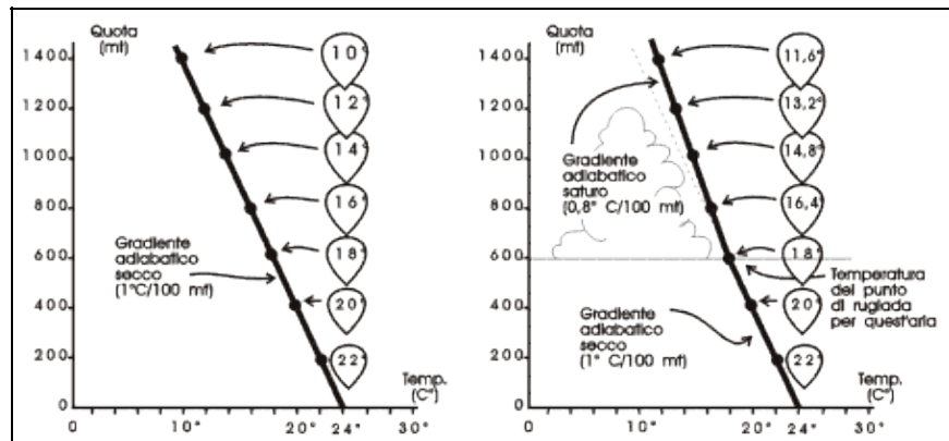
Figura 4-8. I gradienti adiabatici indicano di quanto una massa d'aria, circondata da aria più fredda, si raffredda mentre sale e si espande.
