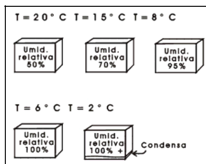
Figura 4-3. L'umidità relativa varia al variare della temperatura.
