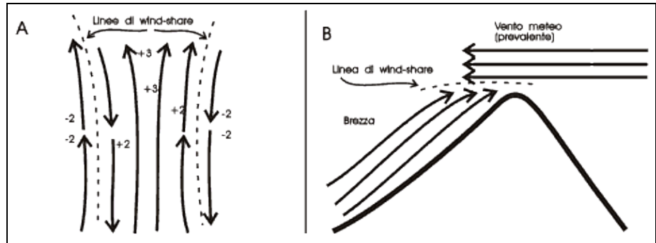
Figura 4-20. A: Wind-shear verticale (ai margini di una termica) . B: wind-shear orizzontale (formato dalla brezza e dal vento prevalente).
