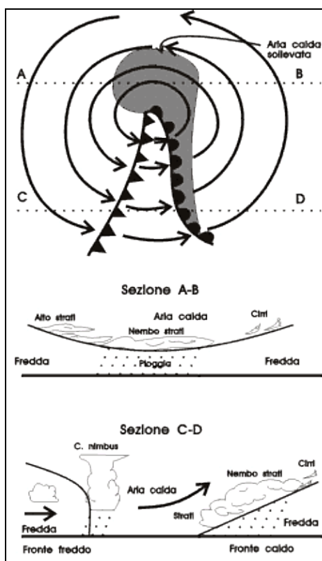
Figura 4-29. Ciclone maturo visto dall'alto e di lato secondo le due sezioni A-B e C-D.
