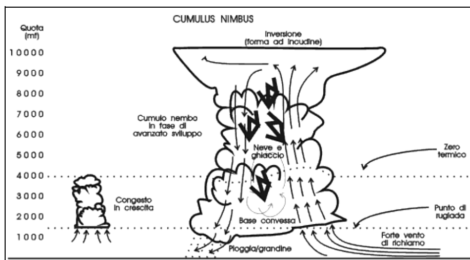
Figura 4-23. Linee di flusso d'aria e dimensioni relative di un Cumulus nimbus: per la forza dei venti ad esso associati e per la notevole turbolenza creata, questa nube viene evitata anche dai grandi aerei di linea.
