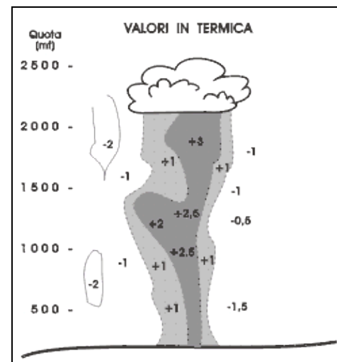
Figura 8-1. Una termica reale: si noti la zona centrale di maggiore ascendenza e la irregolarità della forma.
