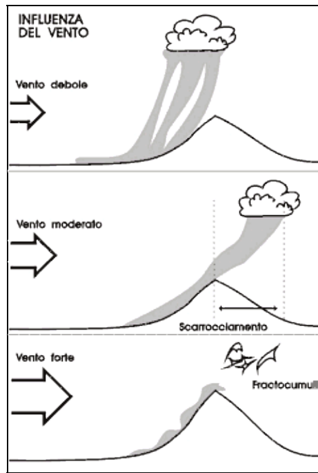
Figura 8-4. Un vento moderato favorisce il distacco delle termiche, uno troppo sostenuto le distrugge.
