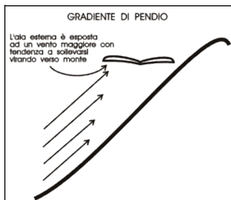
Figura 4–19. Gradiente di vento sul pendio.
