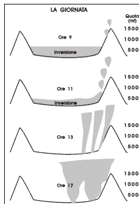
Figura 8–2. A parità delle altre condizioni, la forma delle ascendenze varia di molto, nell'arco della giornata.
