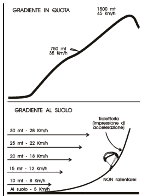
Figura 4-18. Gradienti di vento in quota ed al suolo.
