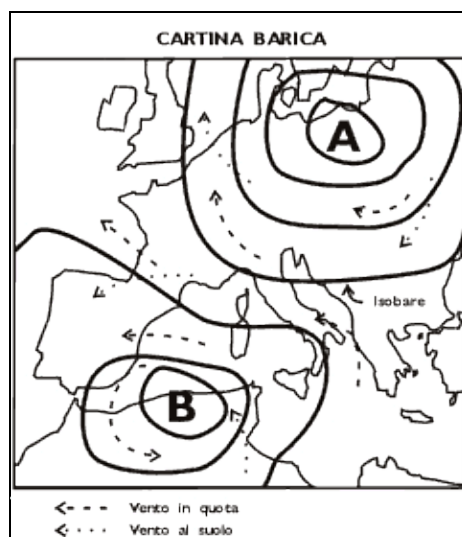
Figura 4-27. Cartina barica: dall'andamento delle isobare è possibile conoscere la direzione dei venti in quota ed al suolo.
