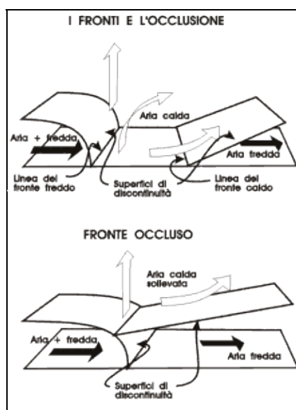
Figura 4-30. Movimenti relativi delle masse d'aria prima e durante l'occlusione.
