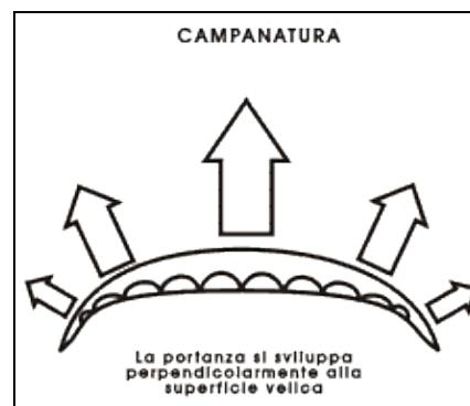
Figura 6–25. Effetto della campanatura sulla direzione delle "linee di portanza": si noti l'effetto di mantenere distesa la parte centrale.
