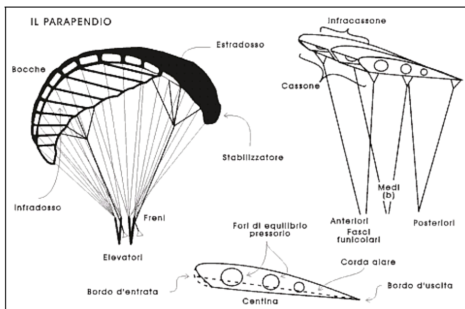
Figura 6-1. Il parapendio e la corretta denominazione delle sue parti.
