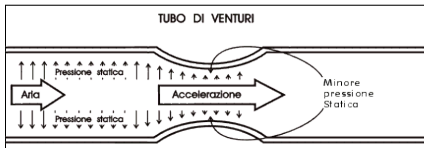
Figura 3-5. Il tubo di Venturi è un tubo con un restringimento: a questo livello l'aria accelera e la pressione statica che essa esercita sulle pareti è quindi minore rispetto al resto del tubo
