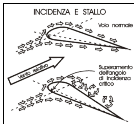
Figura 3–19. Lo stallo si verifica quando i filetti fluidi perdono la loro aderenza e si distaccano dall'estradosso.
