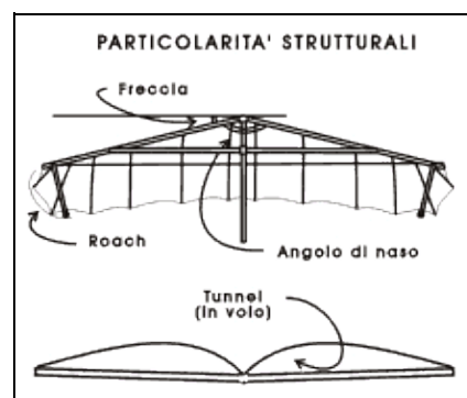
Figura 5-3. Angolo di naso, freccia a roach
