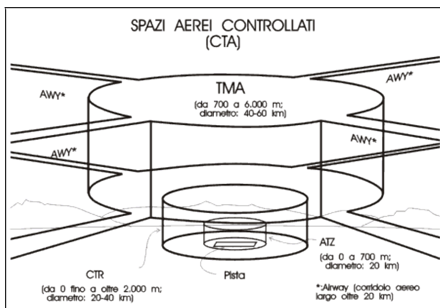
Figura 2.1. Spazi aerei controllati: le AWY confluiscono in un ampio cilindro, sollevato di 700–1000 metri rispetto al suolo, detto TMA. L'aeroporto è "circondato" da due cilindri: uno più piccolo, l'ATZ, ed uno più grande, il CTR.
