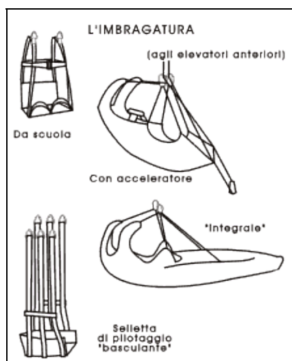
Figura 6-31. Le imbragature disponibili.
