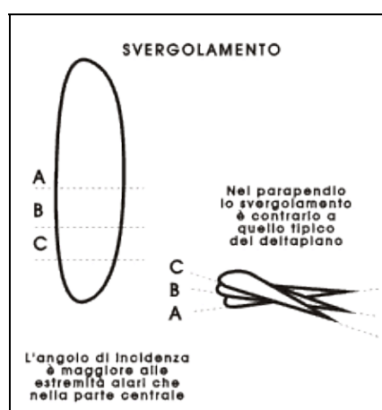
Figura 6-26. Lo svergolamento, presente su alcuni modelli di parapendio, aiuta la riapertura e rende più graduale lo stallo finale.
