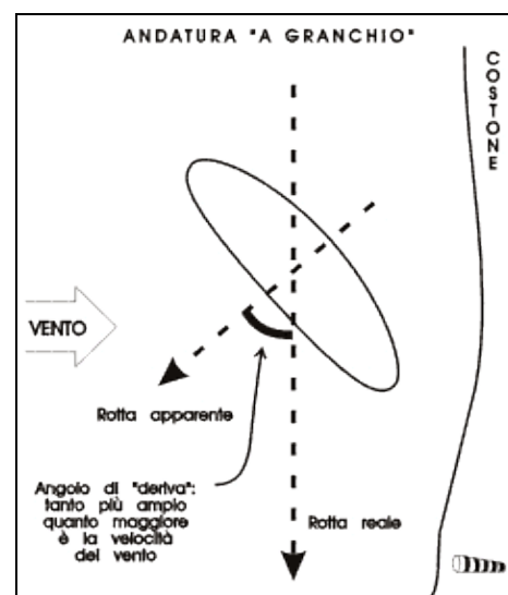
Figura 6-5. Per mantenere una rotta stabilita rispetto al suolo, volando in presenza di vento, è necessario mantenere una rotta apparente tanto più "contro-vento", quanto maggiore è l'intensità del vento stesso.
