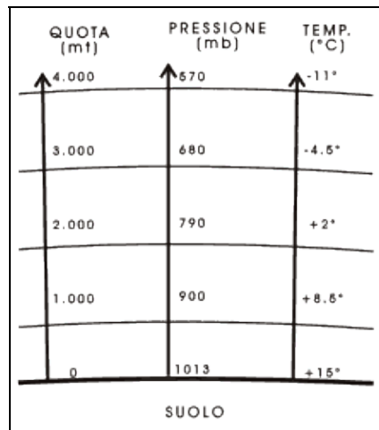
Figura 4-7. Gradiente termico e gradiente barico (pressorio) medi nei primi 4.000 metri di altezza s.l.m.
