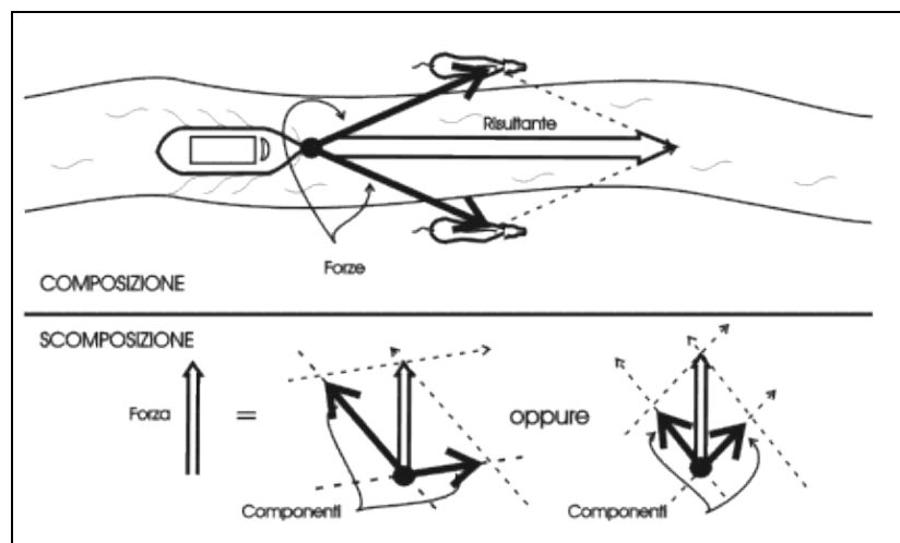
Figura 3-2. Due forze che agiscono nello stesso punto possono venire composte in una sola forza a loro equivalente. Al contrario ogni forza può essere scomposta in altre due con direzioni scelte arbitrariamente.
