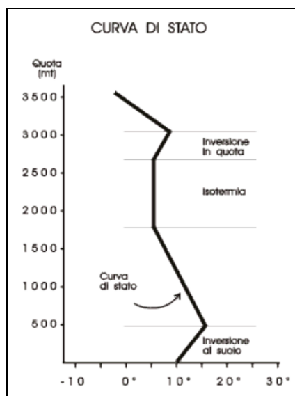
Figura 4-9. La curva di stato indica come varia la temperatura al variare della quota: si notino le inversioni termiche (sia al suolo che in quota). In base alla curva di stato (rilevata giornalmente) è possibile individuare le condizioni di equilibrio dell'aria.
