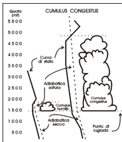
Figura 4-22. Il cumulus congestus, ben più grande dell'humilis, rappresenta una possibile evoluzione verso il cumulus nimbus.
