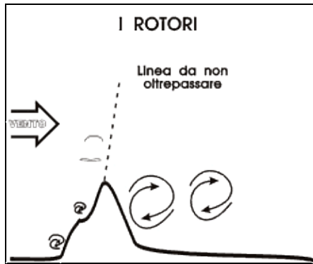
Figura 8-11. I grossi rotori di sottovento e quelli piccoli di sopravvento devono essere attentamente evitati.
