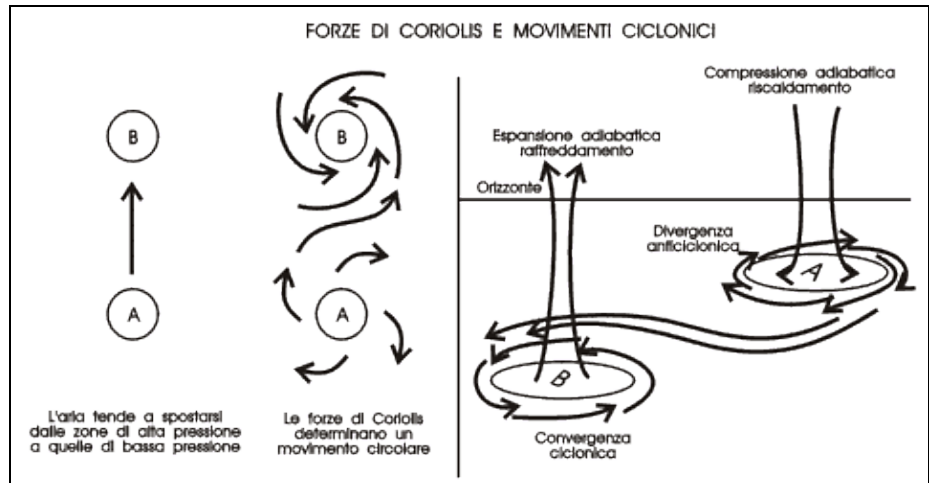
Figura 4-26. L'aria, ruotando, converge verso le zone di bassa pressione (B) e si allontana da quelle di alta pressione (A).
