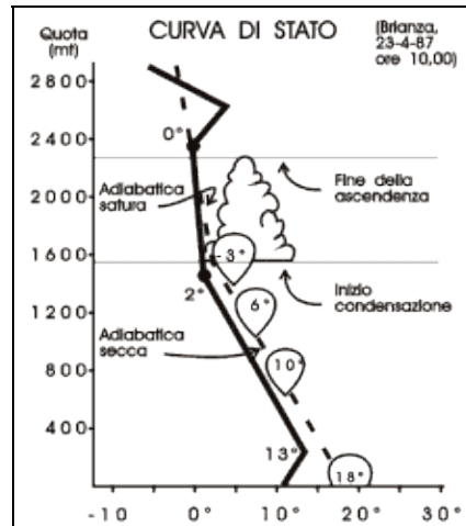
Figura 4-11. Un esempio di curva di stato tratto dalla realtà: Brianza, 23 aprile 1987.
