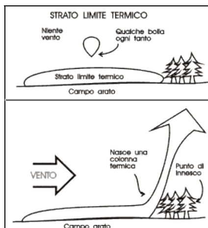
Figura 4-12. Strato limite termico e punti di innesco.
