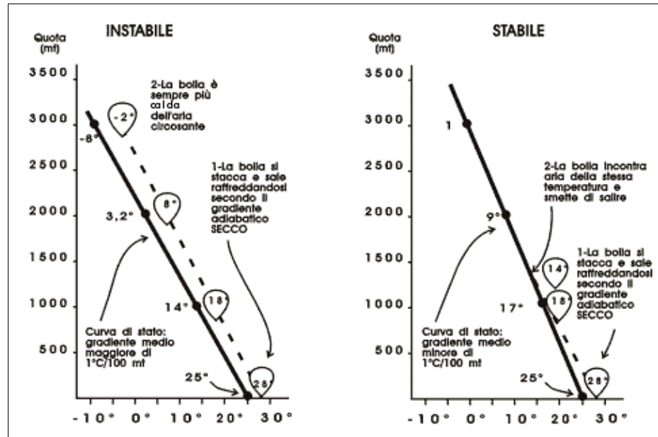
Figura 4-10. Le possibili condizioni di equilibrio dell'aria, deducibili dal confronto tra curva di stato e gradiente adiabatico secco.
