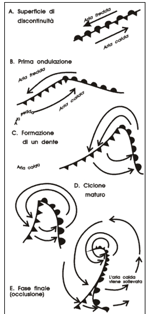
Figura 4-28. I fronti (caldo, freddo ed occluso) compaiono durante le diverse fasi vitali del ciclone: dalla sua genesi (A,B), allo sviluppo e maturità (C,D), alla dissoluzione (E).
