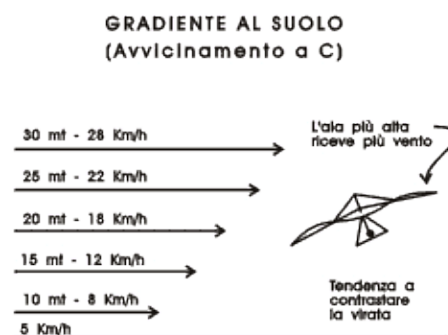
Figura 5-28. Il gradiente di vento (se sostenuto) determina una tendenza a contrastare le ultime virate dell'avvicinamento a C.
