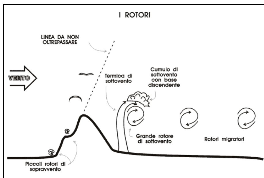
Figura 4-17. I rotori che si formano sottovento ad una montagna possono staccarsi da essa e ritrovarsi anche a diversi chilometri di distanza (rotori migratori); sono da evitare anche i piccoli rotori di sopravvento, tanto più forti quanto più angolato è il "raccordo" tra montagna e pianura.
