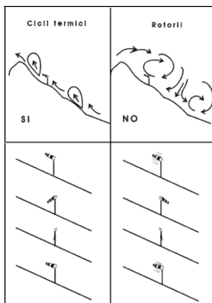
Figura 6-16. È molto importante saper distinguere con sicurezza i cicli termici di pendio da eventuali rotori di sottovento.
