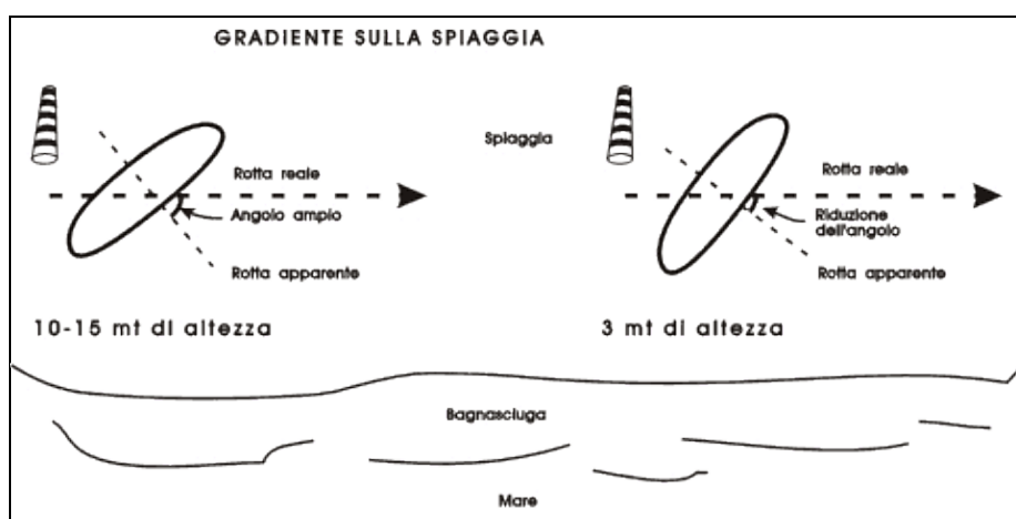
Figura 6-23. Il gradiente di vento su una spiaggia ha il perverso effetto di "attirare" la vela verso l'acqua: per evitare ciò si deve ridurre l'angolo di deriva man mano che ci si avvicina al suolo.
