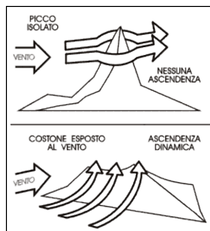
Figura 4-15. Un picco isolato non crea ascendenza dinamica, un largo costone invece si
