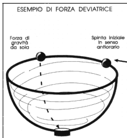
Figura 4-24. Una piccola spinta laterale determina un movimento rotatorio sulla pallina sottoposta alla forza di gravità.
